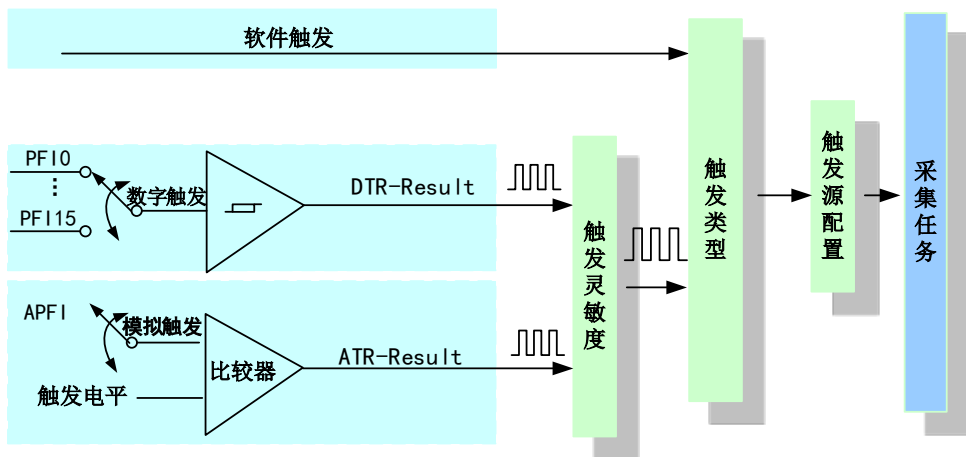
图 6-1-1 触发源选择
