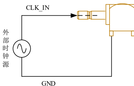
图 4-6-1 时钟输入的连接
