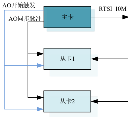
图 4-8-1 主从卡级联
