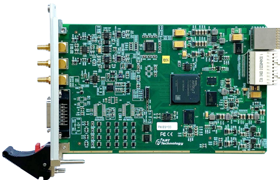
图 3-1-2 PXIe910X 外观图
