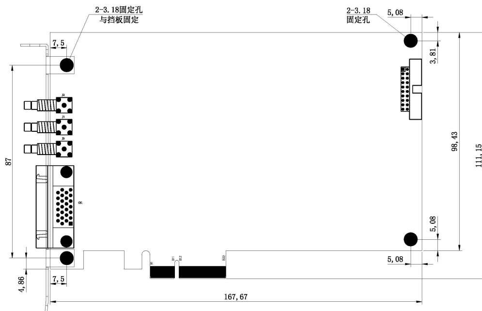
图 3-3-1 PCIe910X 板卡尺寸图
