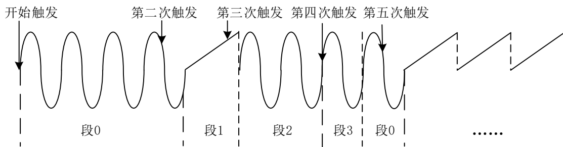
图 6-3-4 突发触发
