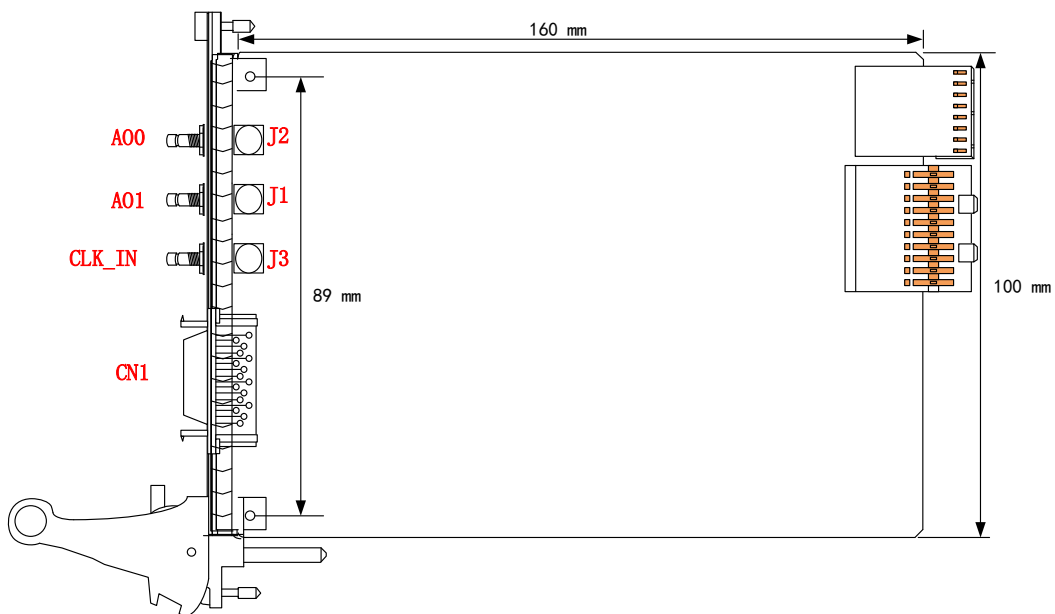
图 3-3-2 PXIe910X 板卡尺寸图
