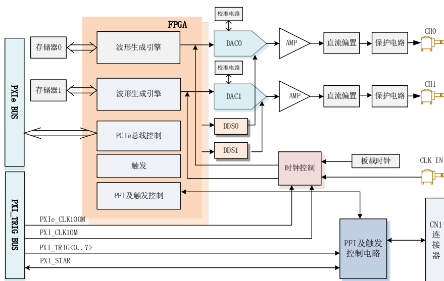
图2-2-2 PXIe910X系统框图
