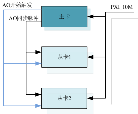
图 4-8-2 主从卡级联
