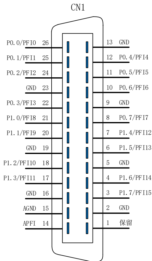
图 3-2-1 CN1 连接器定义
