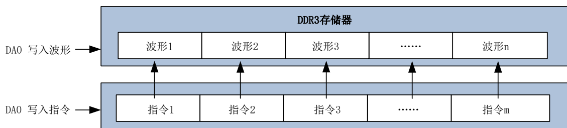
图4-5-1 AO通道存储格式
