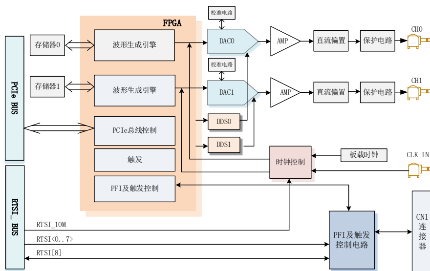
图2-2-1 PCIe910X系统框图
