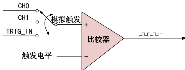
图5-3-2 模拟触发比较器
