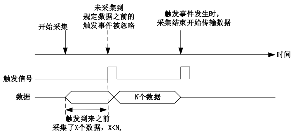
图 4-8-1-5 预触发--采集数据小于 N
