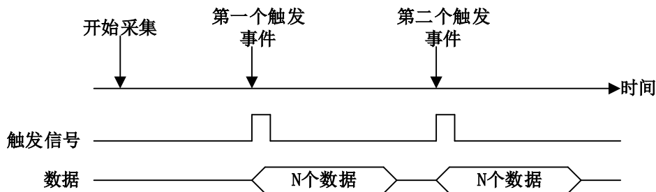
图 4-8-1-7 后触发和延时触发的重复触发
