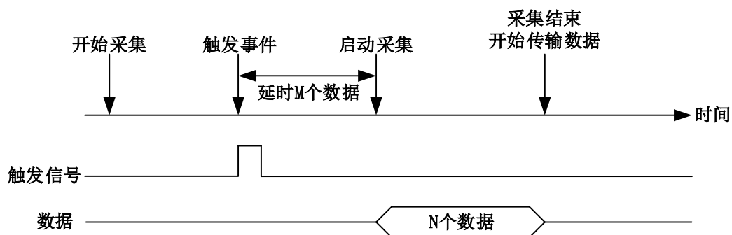
图 4-8-1-6 硬件延时触发
