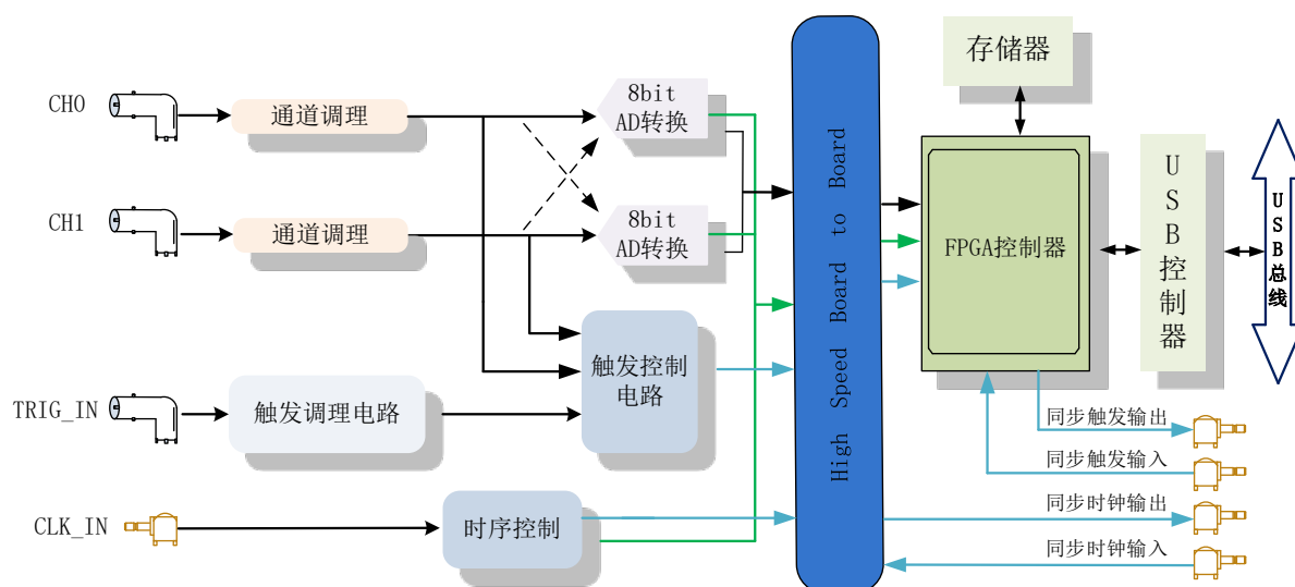
图 3-1-1 USB8910N 系统框图
