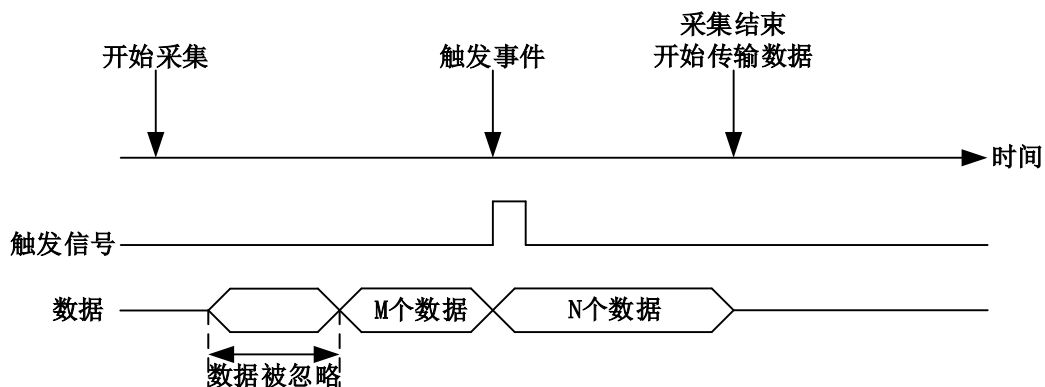
图 4-8-1-2 中间触发
