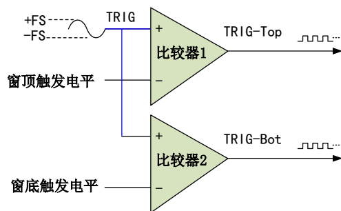
图5-3-4 比较器
