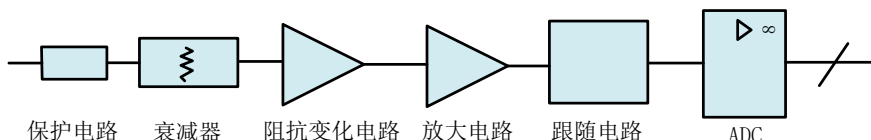
图 4-1-1 AI 功能框图
