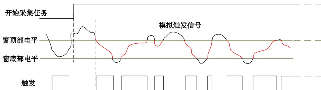
图5-3-5 模拟窗触发--入窗
