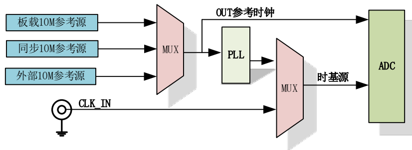
图 4-7-1 时基源框图
