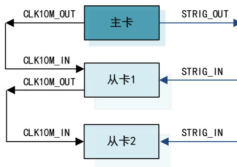
图4-9-1 主从卡级联
