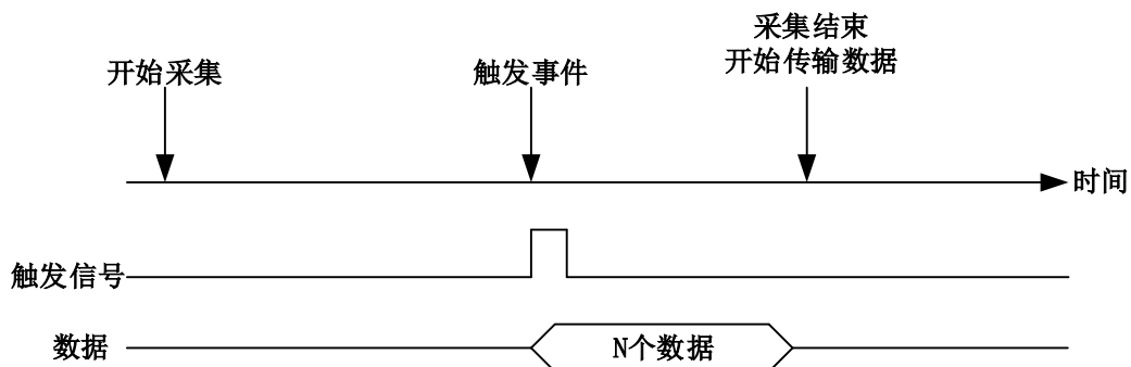
图 4-8-1-3 后触发
