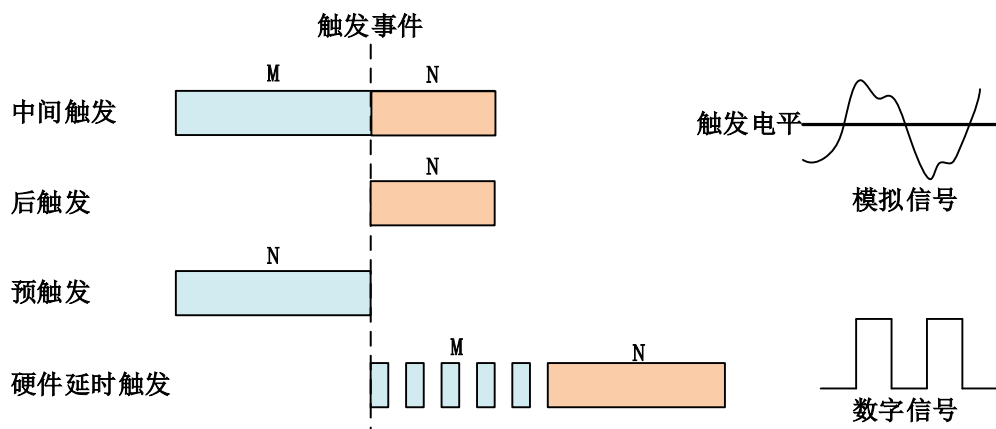
图 4-8-1-1 AI 触发模式
