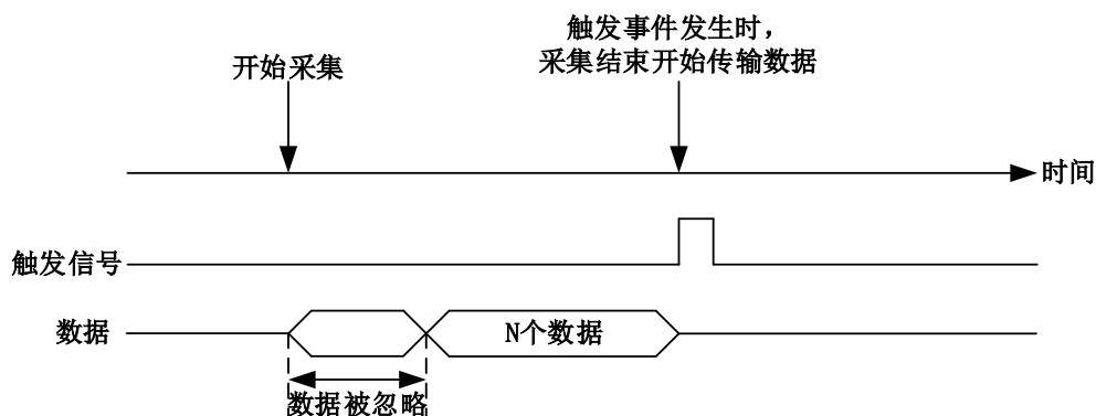
图 4-8-1-4 预触发
