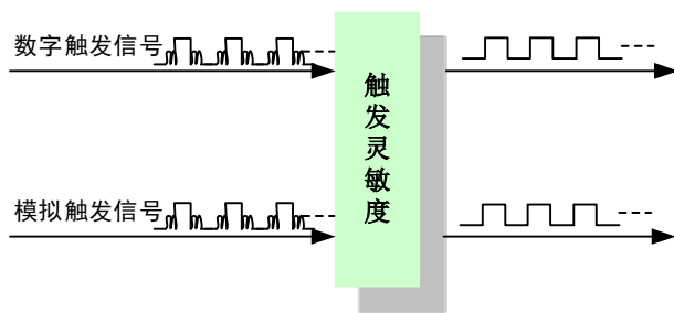
图 8-3-1 触发灵敏度
