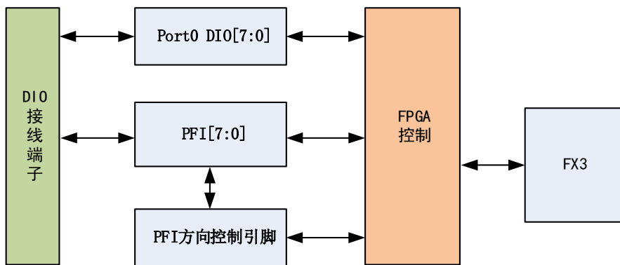
图7-1-1 DIO功能框图
