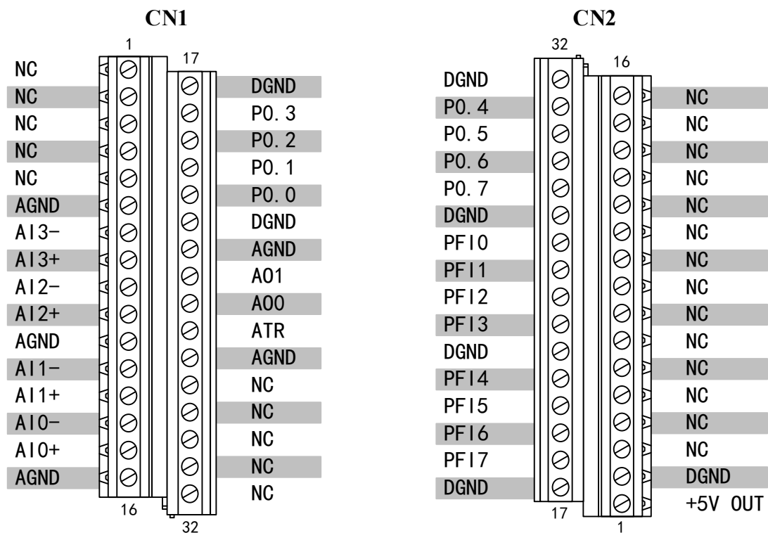
图 3-2-1 接线板管脚定义
