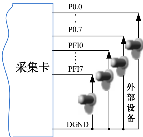
图7-2-1 DI 数字量输入的连接
