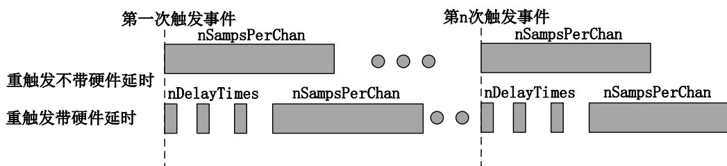
图 8-2-5 AI 重触发
