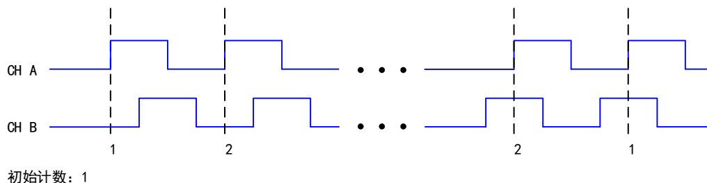
图 6-7-1 X1 编码
