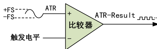
图8-3-4 模拟触发比较器
