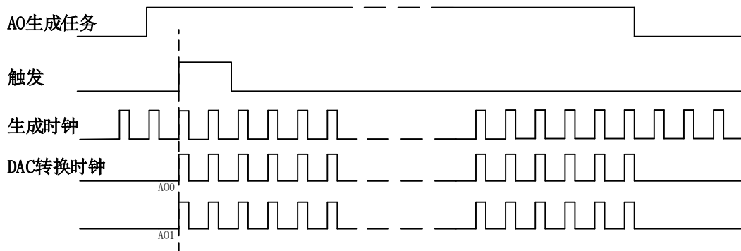
图5-7-3 内、外时钟连续采样
