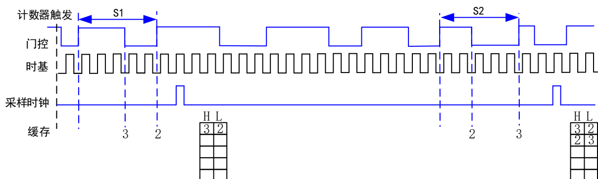
图 6-4-3 采样时钟缓冲脉冲测量
