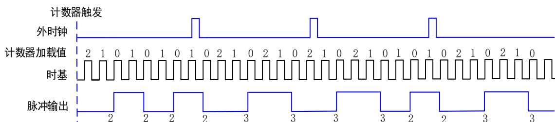
图 6-8-8 有限缓冲外时钟脉冲序列生成
