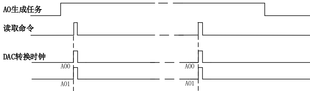
图5-7-1 按需单点采集
