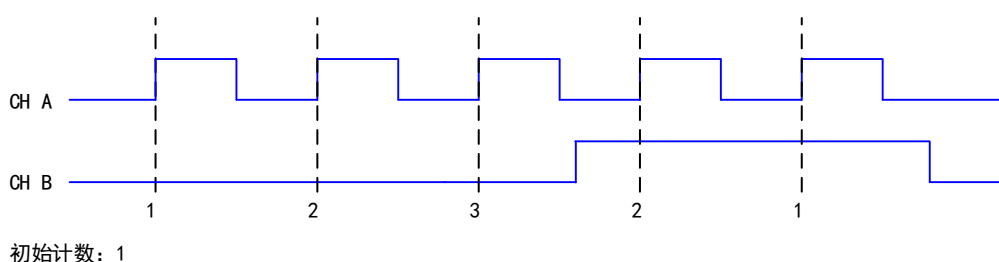
图 6-7-5 单脉冲编码
