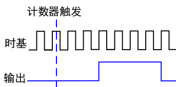
图 6-8-1 单脉冲生成
