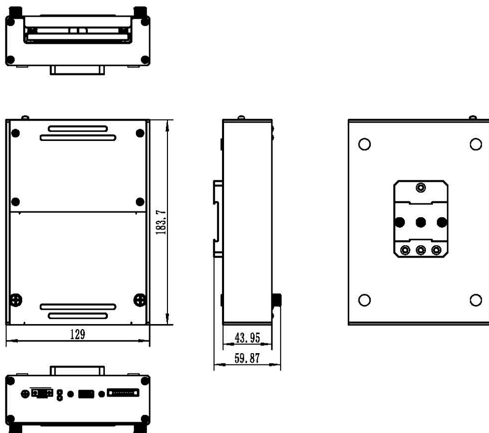
图 3-3-1 ART-D5027 外壳尺寸图
