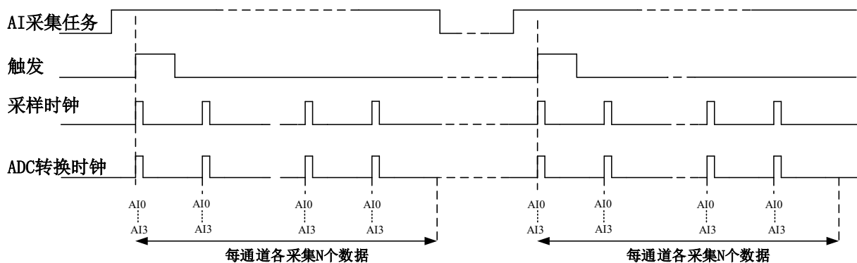
图 4-7-2 有限点采样
