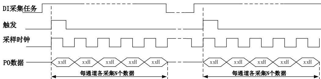
图 7-5-2 有限点采样
