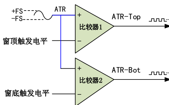
图8-3-6 比较器
