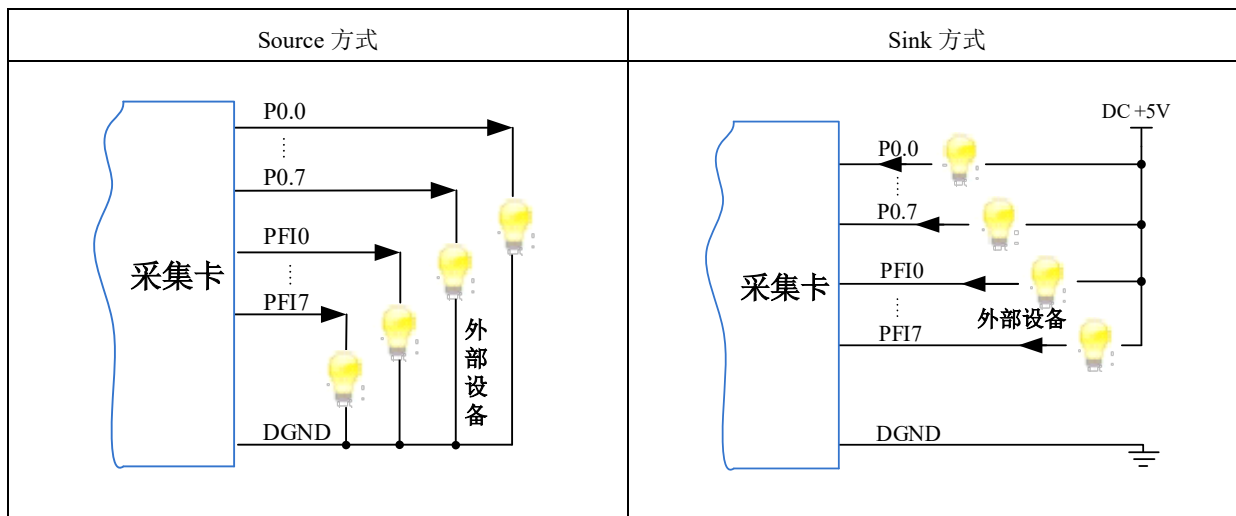
图7-3-1 DO 数字量输出的连接
