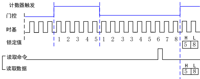
图 6-4-1 单（按需）脉冲测量
