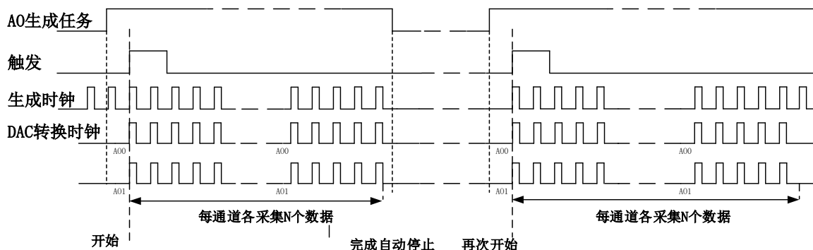
图5-7-2 内、外时钟有限点采样
