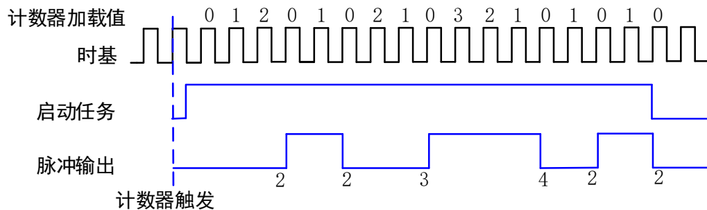
图 6-8-7 有限隐式缓冲脉冲序列生成
