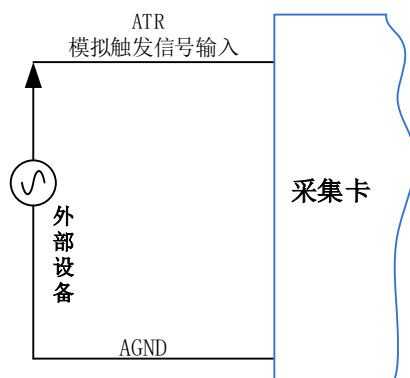
图8-3-3 模拟触发连接方法
