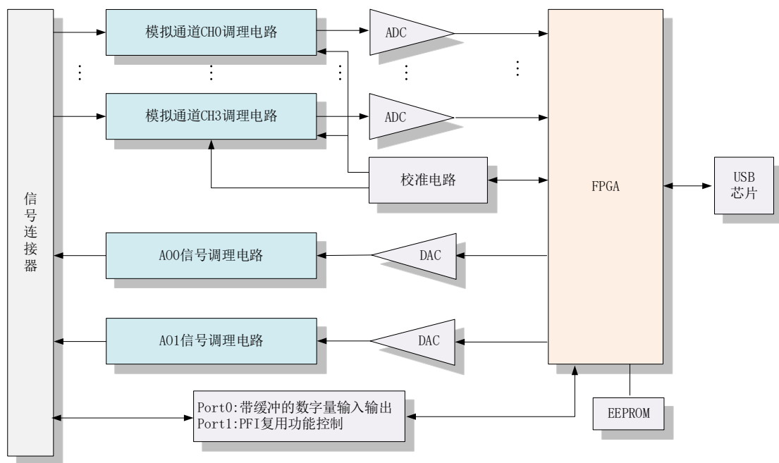
图2-2-1 ART-D5027系统框图
