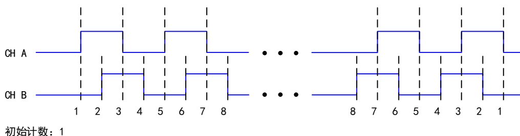
图 6-7-3 X4 编码
