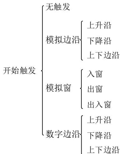
图 8-2-1 开始触发分类
