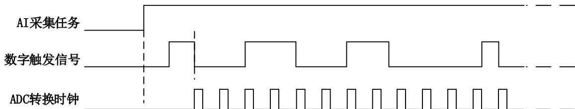
图 8-2-2 数字触发--下降沿触发
