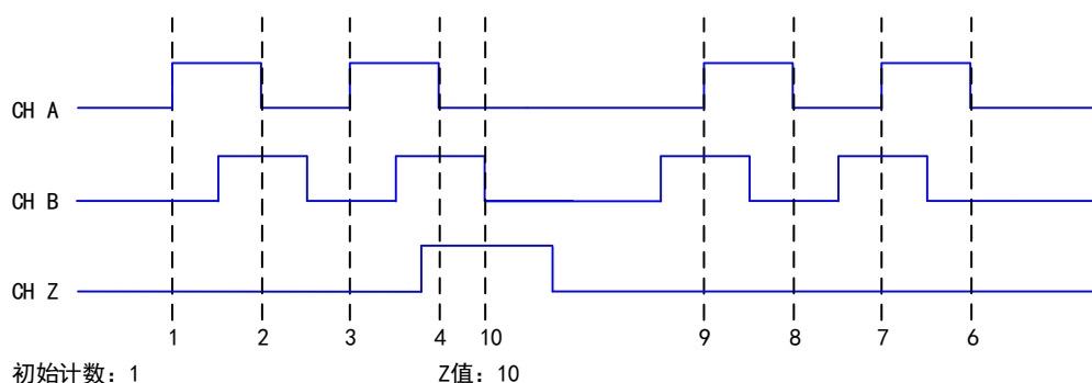
图 6-7-6 Z 索引
