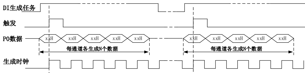
图7-6-2 有限点生成
