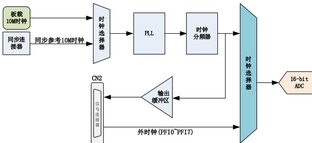
图 4-6-1 AI 时钟结构框图
