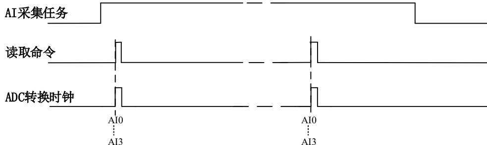
图4-7-1 按需单点采集
