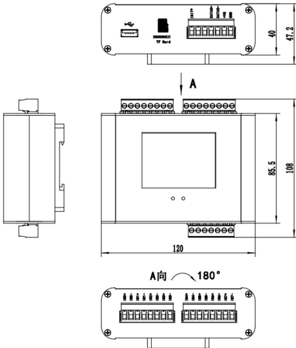
图 2 MDQ-8001URM 产品尺寸图
