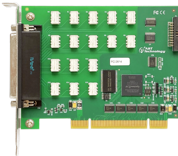
图 3-1-1 PCI2614 外形图
