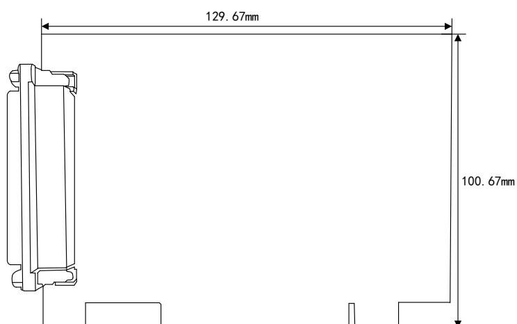
图 3-1-1 PCI2614 尺寸图
