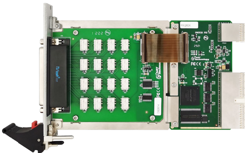
图 3-1-2 PXI2614 外形图
