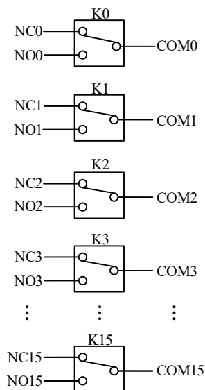
图 2-2-1 硬件框图
