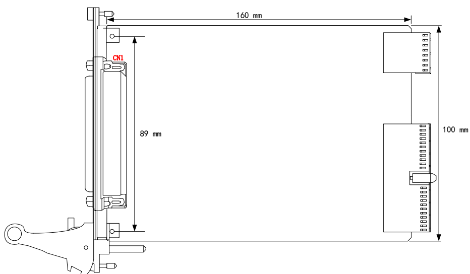
图 3-1-4 PXI2614 尺寸图
