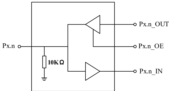
图6-1-1 DIO功能框图
