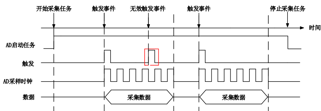
图 7-2-6 重触发
