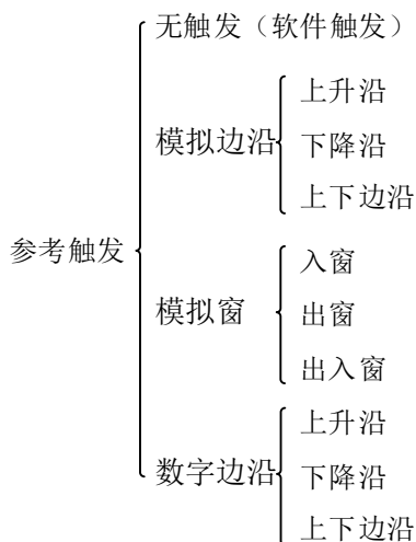
图 7-2-7 参考触发分类
