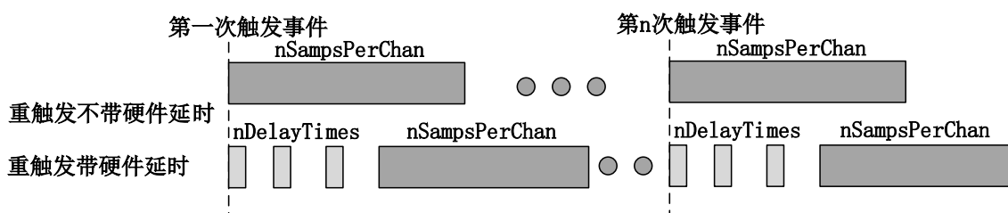
图 7-2-5 AI 重触发
