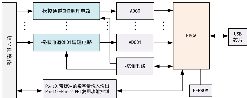
图2-2-1 USB2888系统框图
