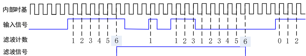
图 5-9-1 数字滤波
