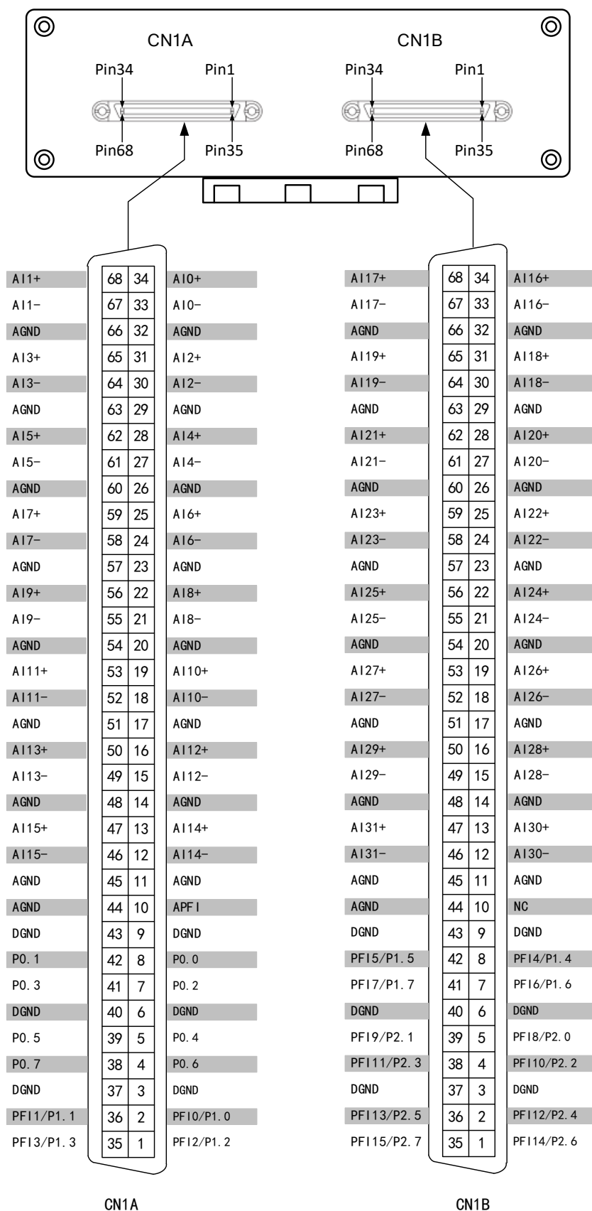
图3-2-2 USB288X-V 管脚定义
