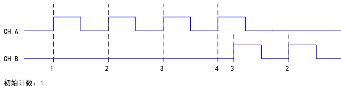
图 5-7-4 双脉冲编码
