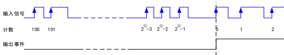
图 5-10-2 反转方式输出
