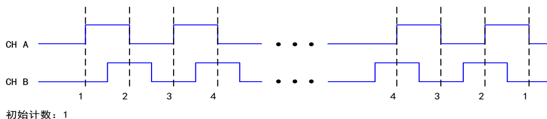
图 5-7-2 X2 编码
