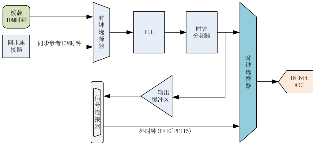
图 4-6-1 AI 时钟结构框图
