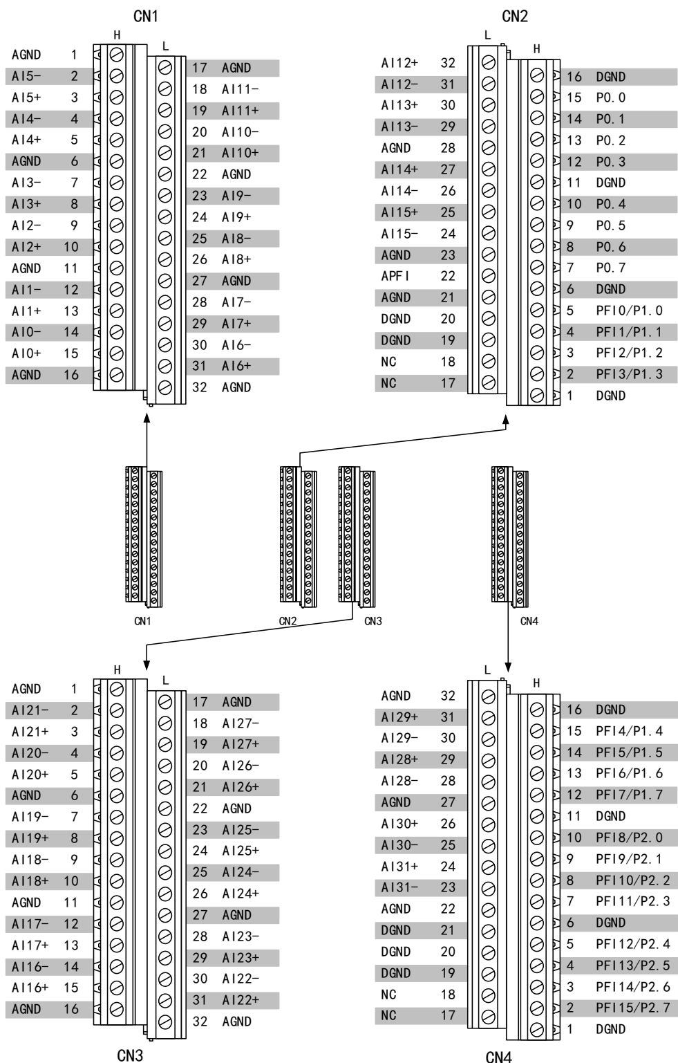
图 3-2-1 USB288x-D 管脚定义
