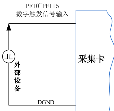
图7-3-8 数字触发连接方法
