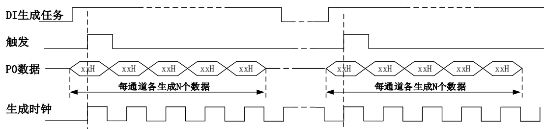
图6-6-2 有限点生成
