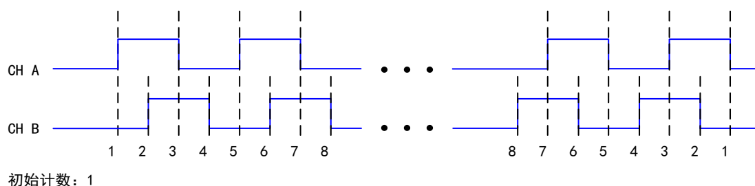
图 5-7-3 X4 编码
