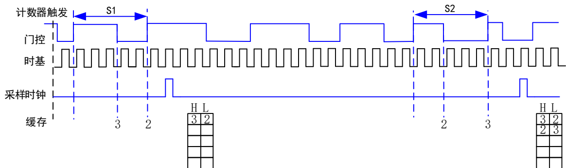
图 5-4-3 采样时钟缓冲脉冲测量
