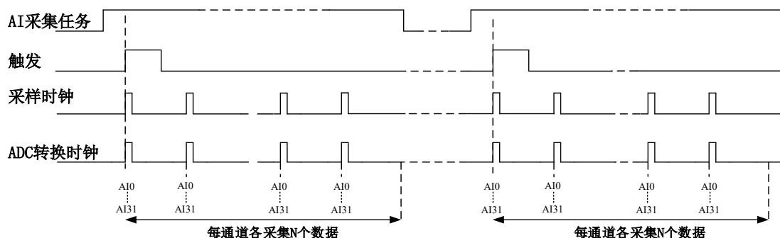
图 4-7-2 有限点采样
