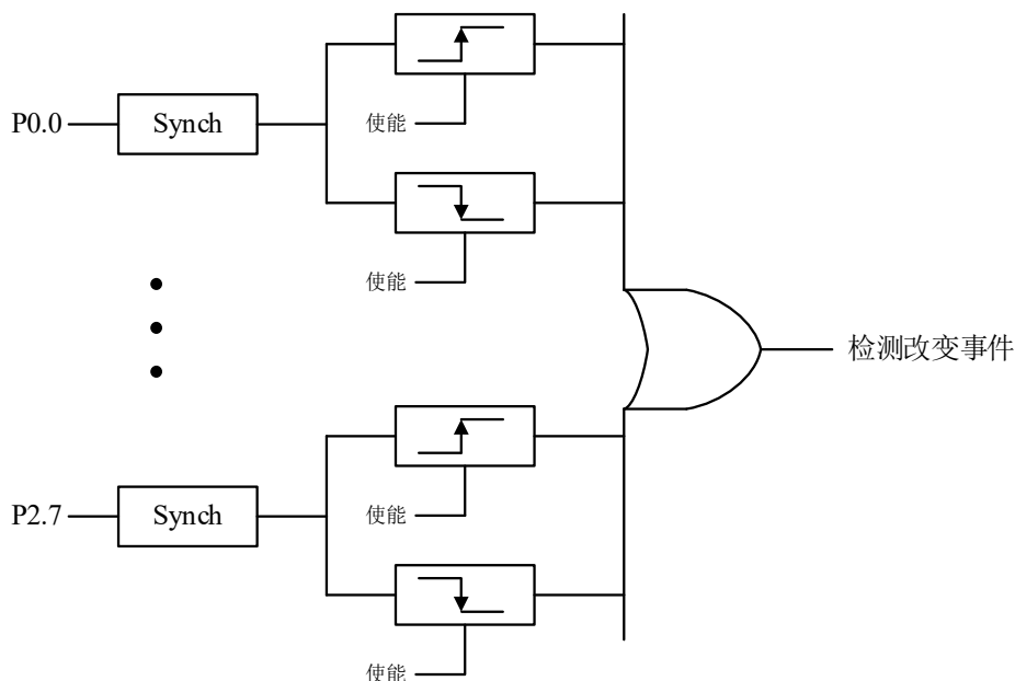
图 6-8-1 检测改变电路框图
