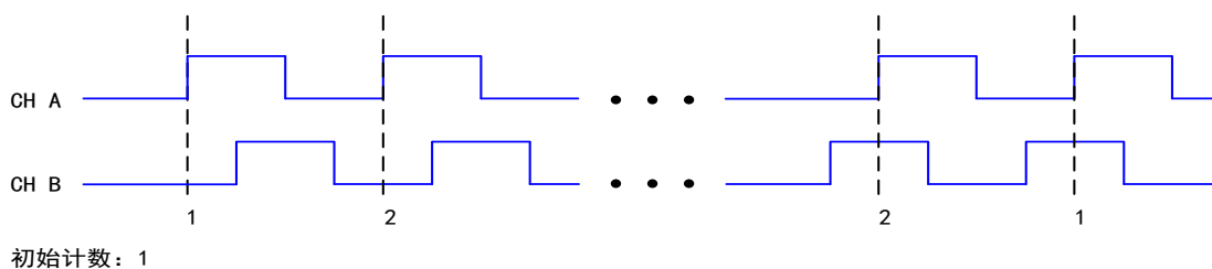
图 5-7-1 X1 编码
