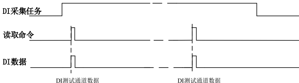
图6-5-1 按需单点采集
