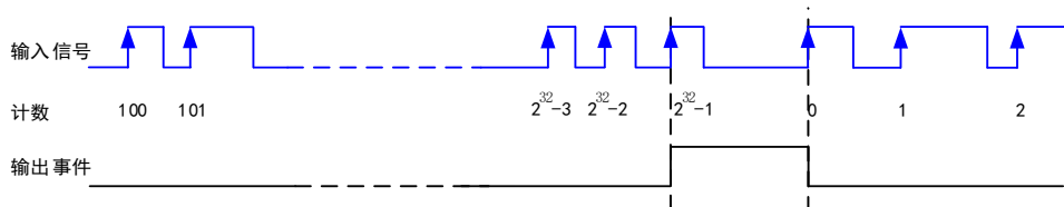
图 5-10-1 脉冲方式输出
