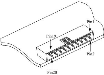
图 3-2-3 RTSI 的 Pinout 图
