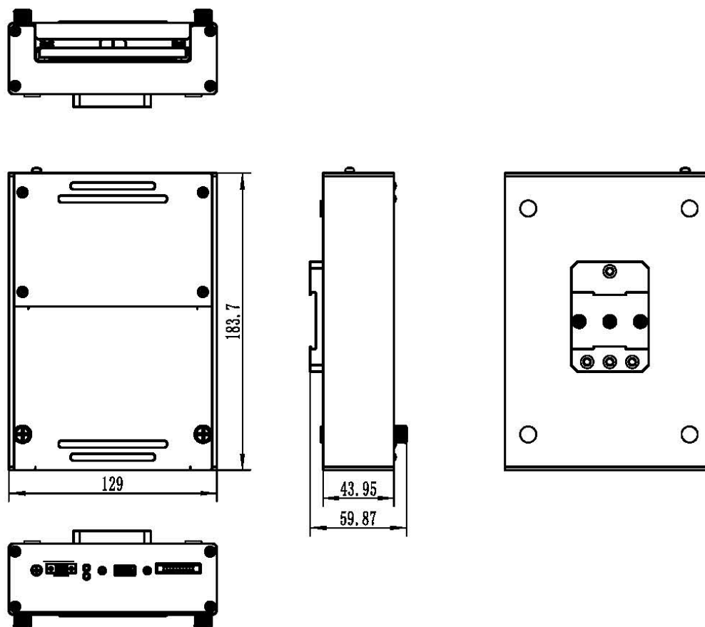
图 3-3-1 USB288x 外壳尺寸图
