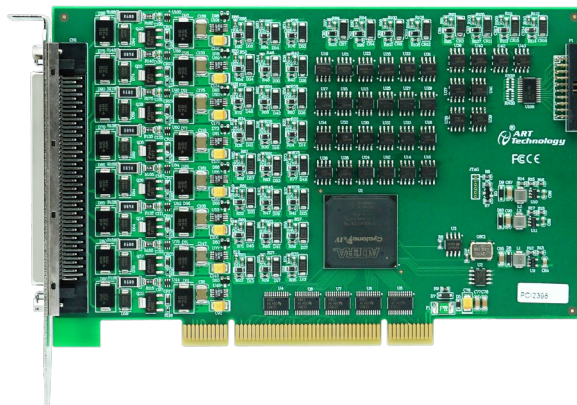
图 3-1-1 PCI2398 正面图
