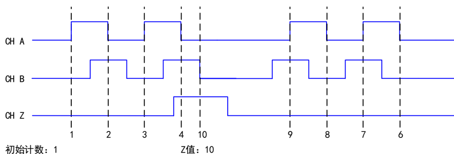
图 4-7-6 Z 索引
