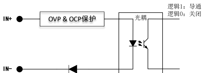
图 3-4-1 输入端电路
