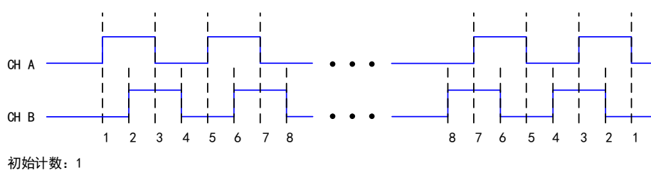
图 4-7-3 X4 编码
