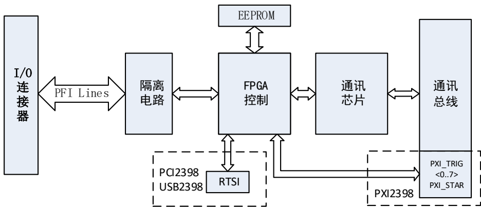
图2-2-1 2398系统框图
