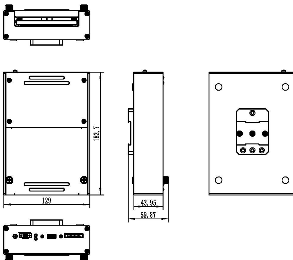
图 3-2-4 USB2398 外壳尺寸图
