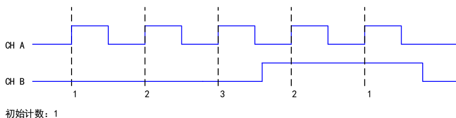
图 4-7-5 单脉冲编码
