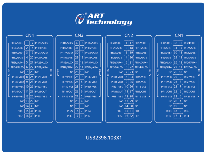
图3-3-2 USB2398 螺栓端子管脚定义
