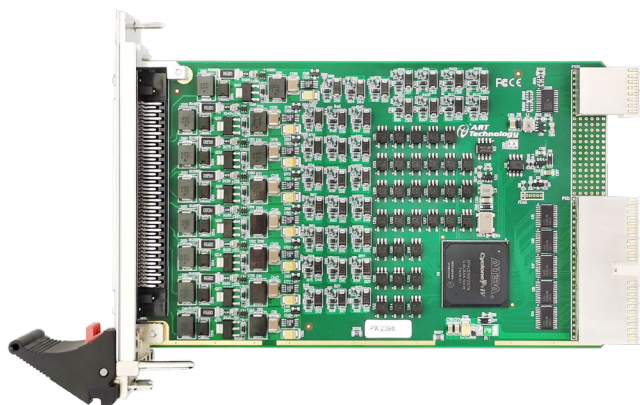
图 3-1-2 PXI2398 正面图
