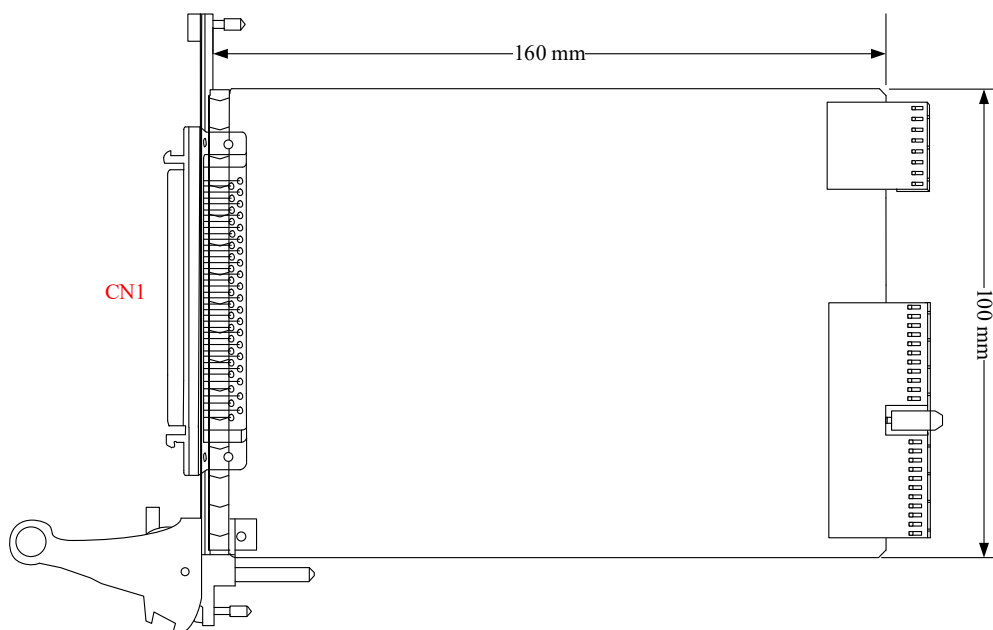
图 3-2-2 PXI2398、CPCI2398 板卡尺寸图
