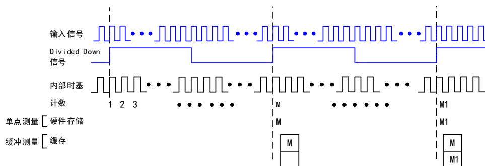
图 4-2-3 大范围信号频率测量上升沿有效示意图
