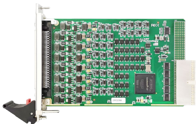
图 3-1-3 CPCI2398 正面图
