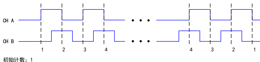
图 4-7-2 X2 编码
