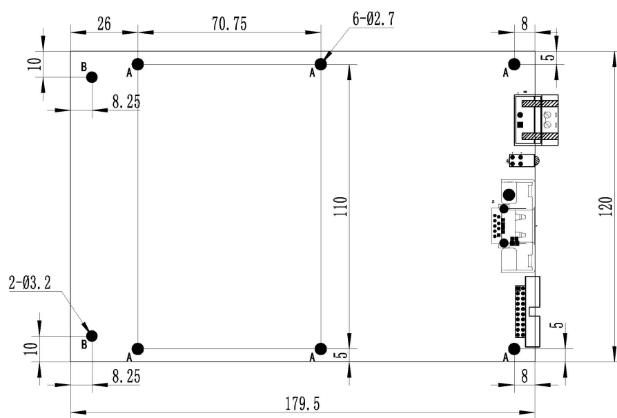
图 3-2-3 USB2398 板卡尺寸图
