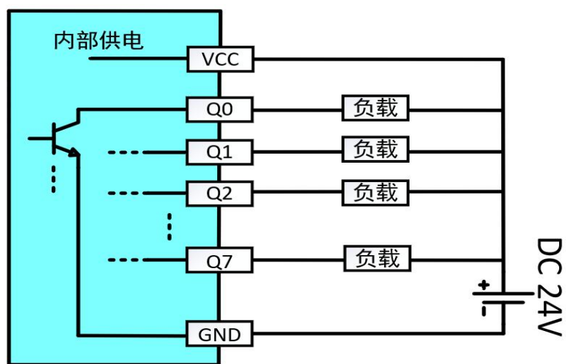
图 3 输出接线
