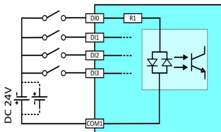
图 2 输入接线
