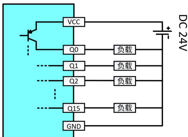
图 2 输出接线
