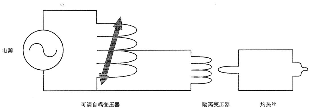
图 2 试验电路
