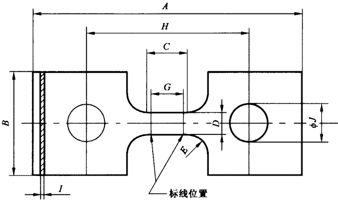
图 3 类型 3 试样
