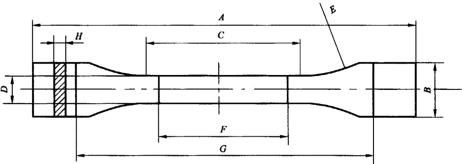
图 1 类型 1 试样
