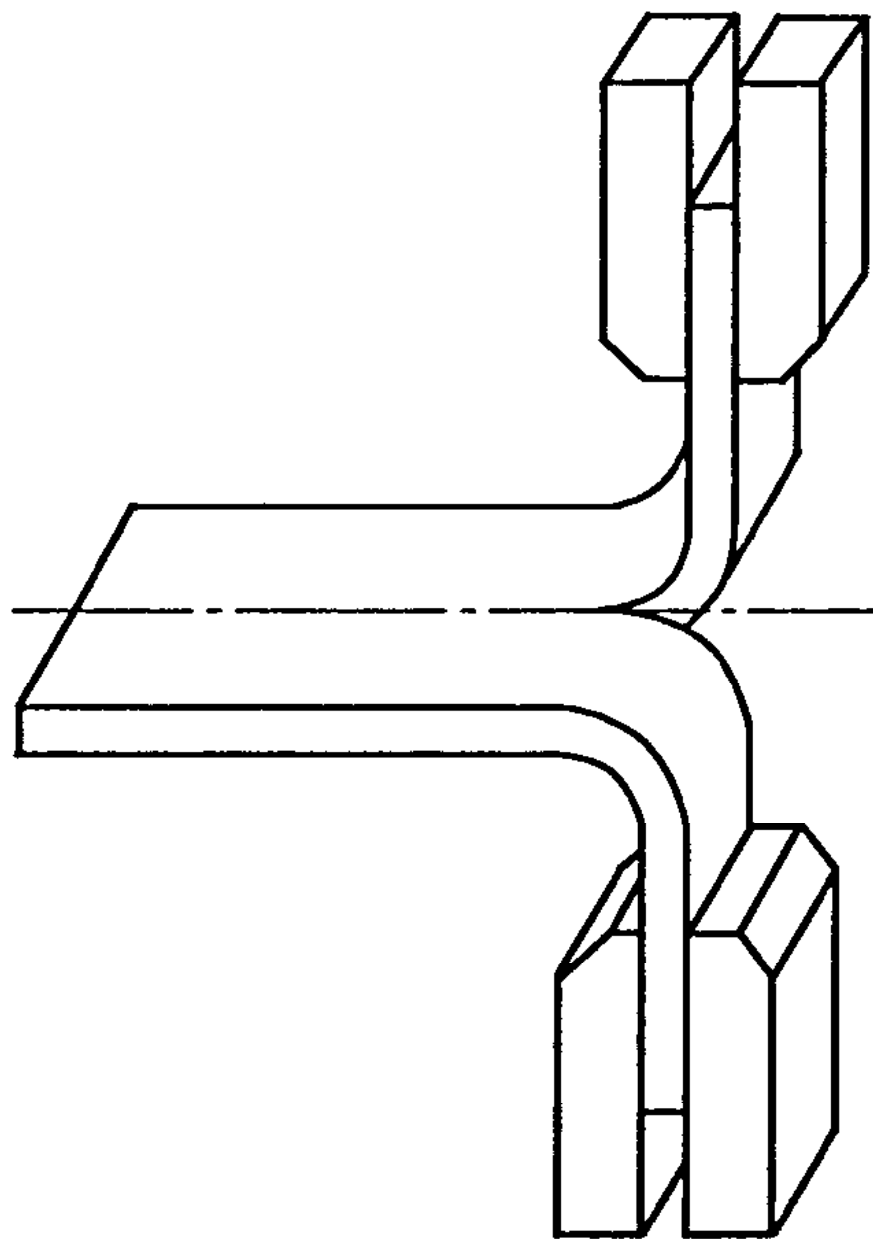
图4 在拉力试验机上裤形试样的状态
