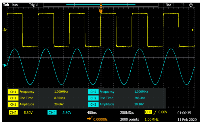
图5: 测量值是透明的，因此不会挡住波形
