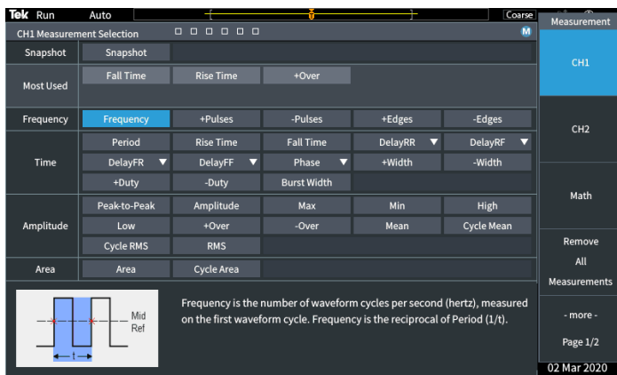
图4: 在一个屏幕上列出和选中所有测量
