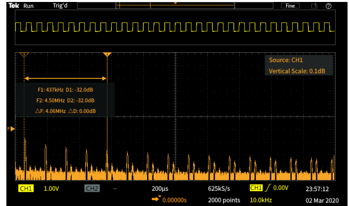
图6: 时域源波形可以显示在 FFT 频率频谱上方
