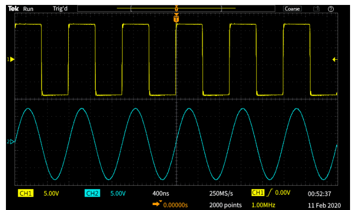
图3: 在缩放模式下，显示屏上半部分显示整个记录的概况，下半部分显示详细的放大后视图。
