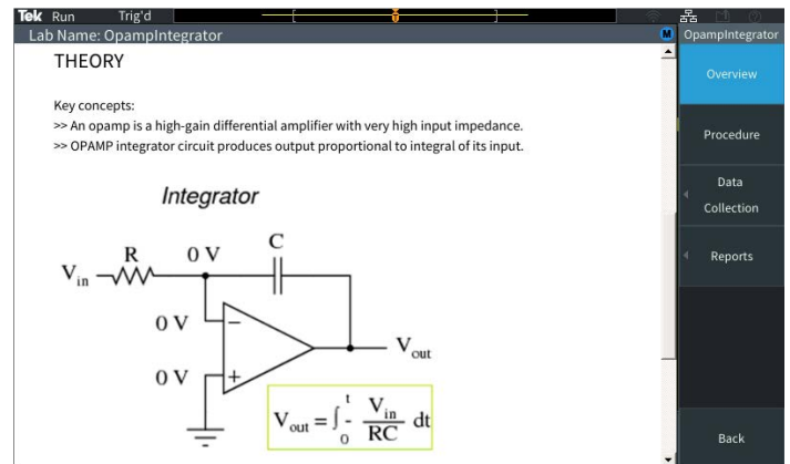
图 10: 课件功能允许学生在仪器显示器上查看实验信息
