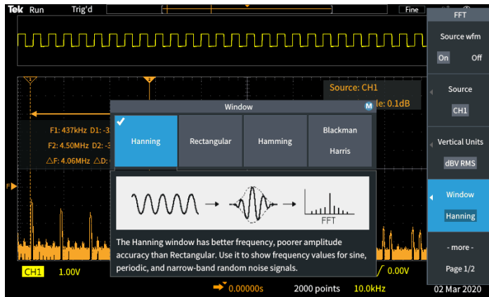
图 7: HelpEverywhere® 小贴士解释了重要设置。
