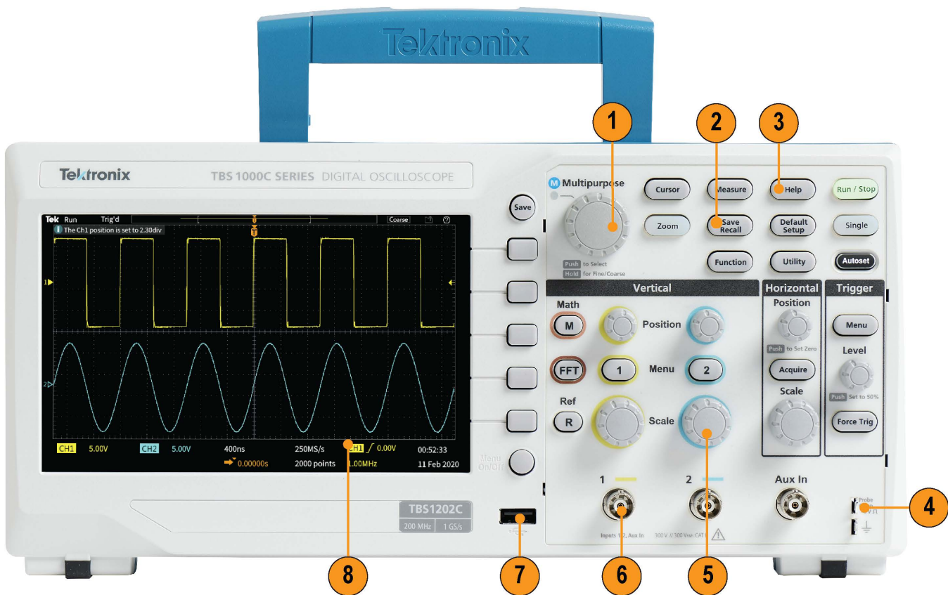
图1: TBS1000C 前面板
