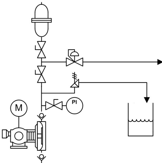
图3：吐出管路
