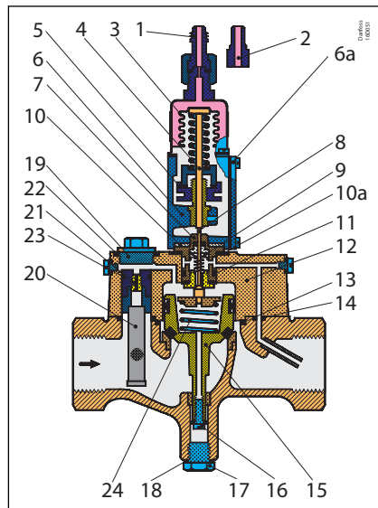
图 4: WVS 40
