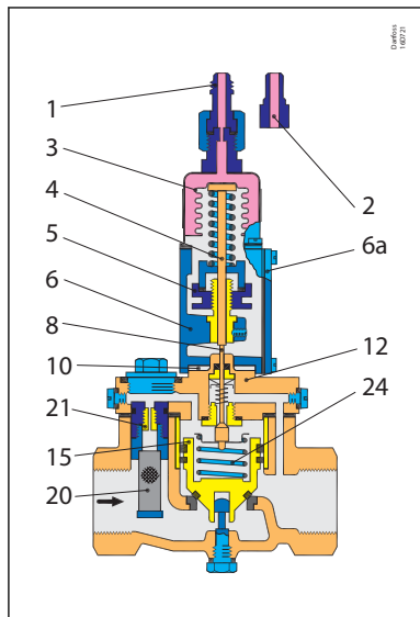
图 3: WVS 32
