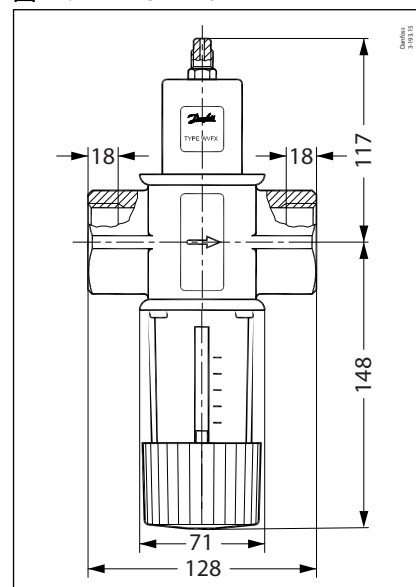
图 11: WVFX 32 – 40
