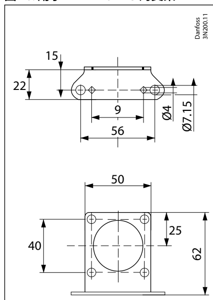
图 10: 用于 WVFX 10 – 25 的支架
