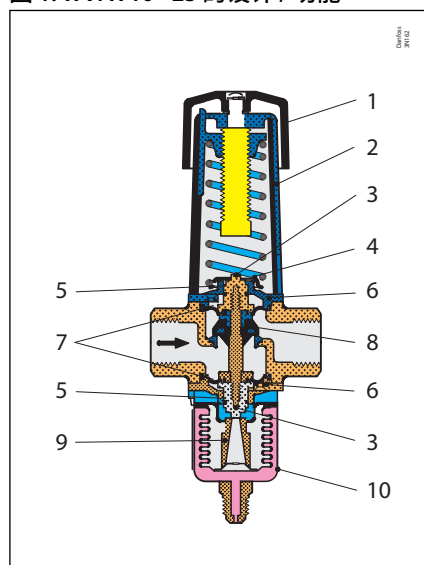
图 1: WVFX 10 - 25 的设计 / 功能
