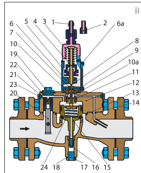
图 5: WVS 50 - 100
