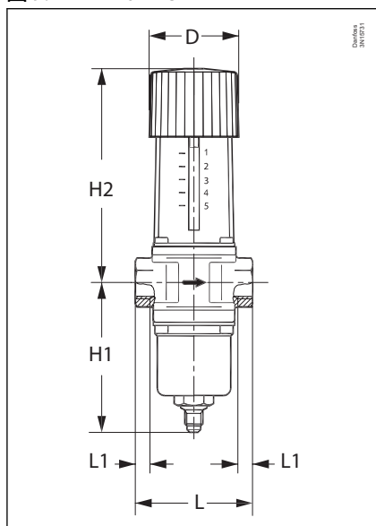
图 9: WVFX 10 – 25
