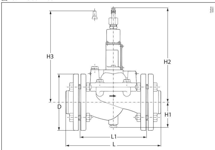
图 13: WVS 50 – 100
