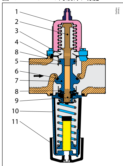
图 2: WVFX 32 - 40 的设计 / 功能
