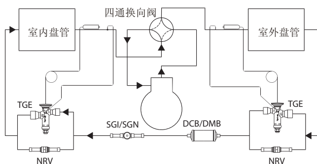
图6. 常规冷暖两用热泵型空调机组系统
