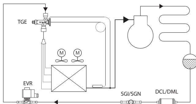
图5. 传统制冷系统
