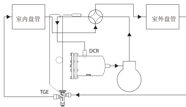
图7. 简化后的冷暖两用热泵型空调机组系统
