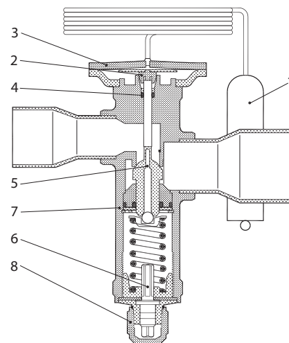
图3 平衡流口设计 双向流过热度可调
