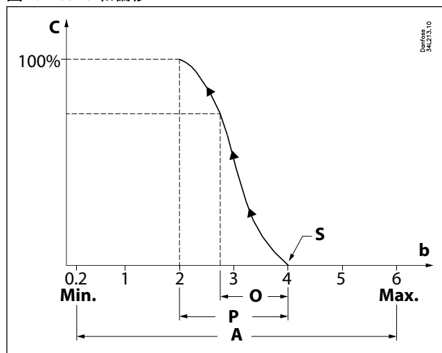
图 2: P-band 和偏移
