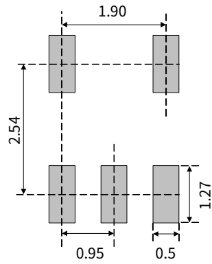
SOT-23-5/TSOT-23-5
