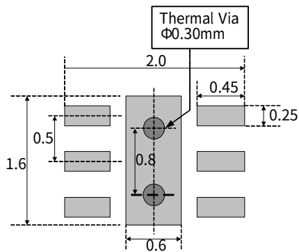
TDFN1.6x1.6-6
